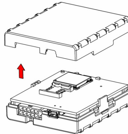
② Remove GE-AM ECO case
